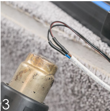
Schrumpfschläuche über die Lötstelle ziehen und mit Heißluftfön erwärmen, bis diese sich ganz zusammen gezogen haben.
